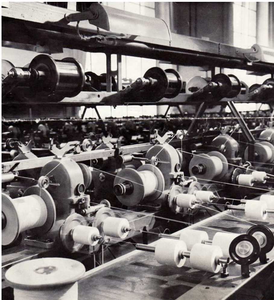
Fig. 12 – Pfäffikon, fabbrica Huber: macchinari per il rivestimento dei fili di rame (materiale di Rita Ropelato)
